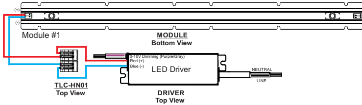
One Module Wiring (1P)
